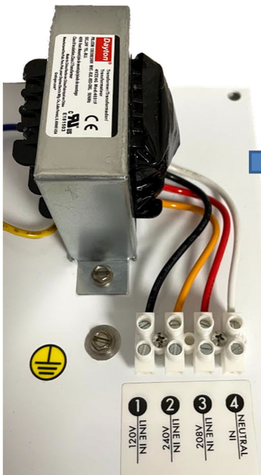
Original Transformer PN 4510157
